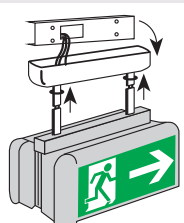
Stropná konzola s predĺžením 0,5 m
